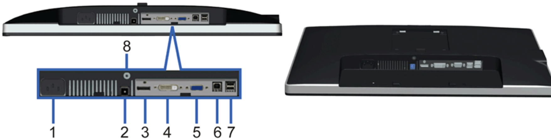
底視圖
